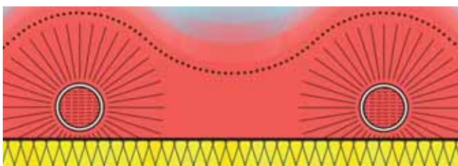
Standard Fußbodenheizung
